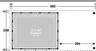
Eleganto 3024 mit Seitendach 280 cm rechts
