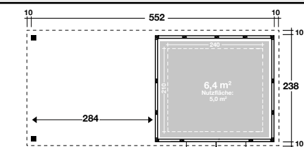
Eleganto 2724 mit Seitendach 280 cm links
